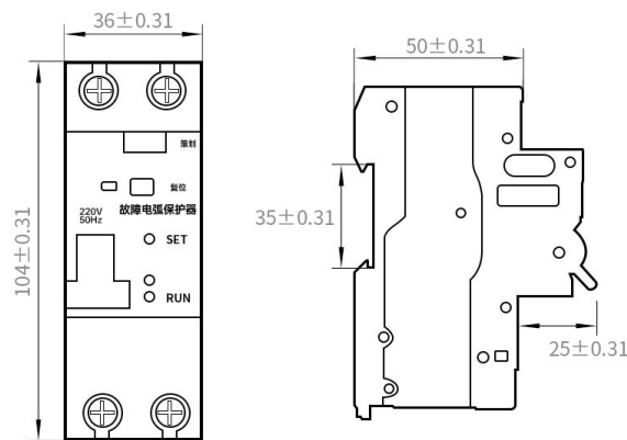
图 3 外形及安装尺寸
